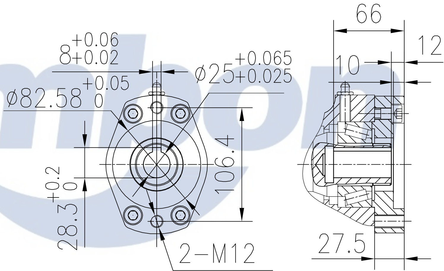
B向视图
