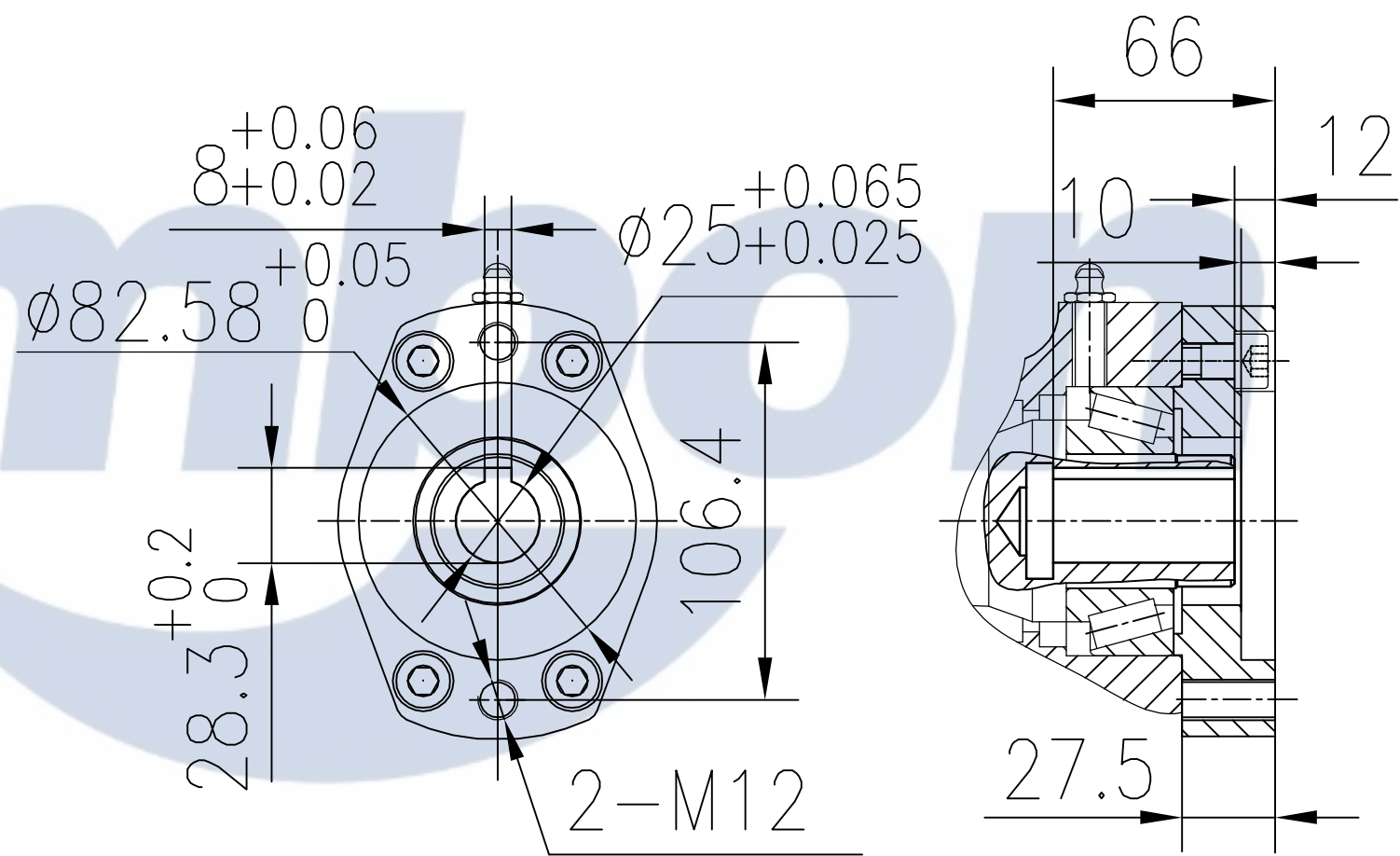
B 向视图
